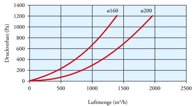
Druckverlust und Luftmenge (Länge: 3 m)
